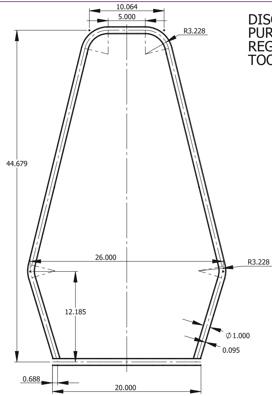
SECTION D-D
